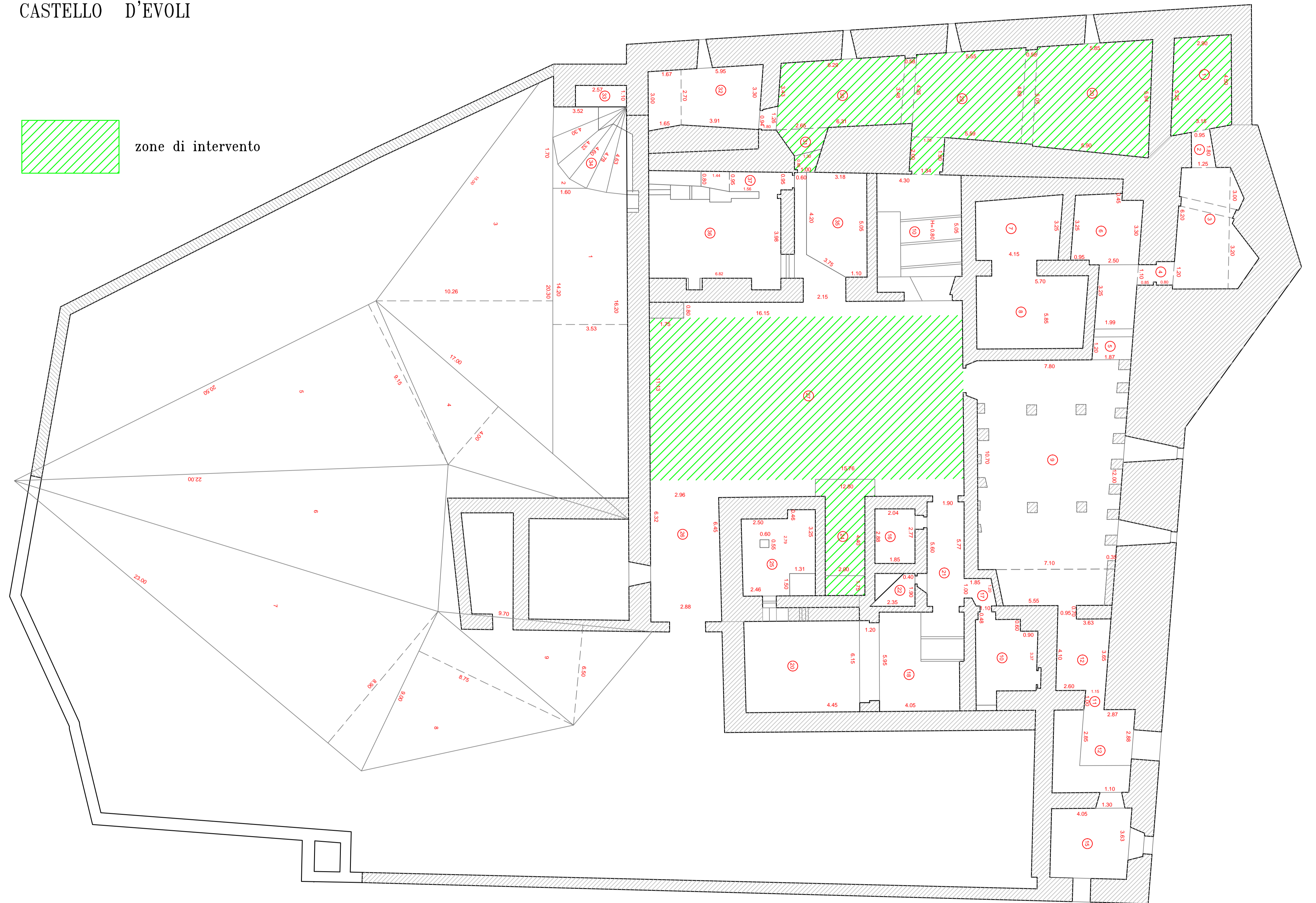
Pianta strutture emergenti
